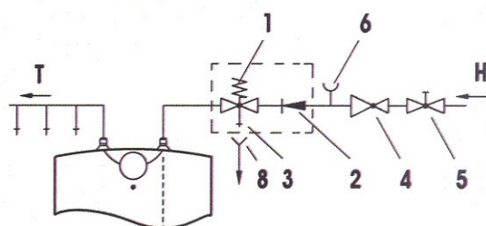
Provedení pod odběrné místo
