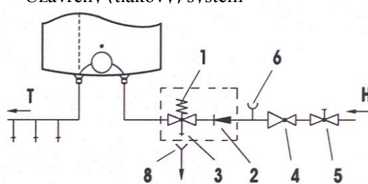
Provedení nad odběrné místo
